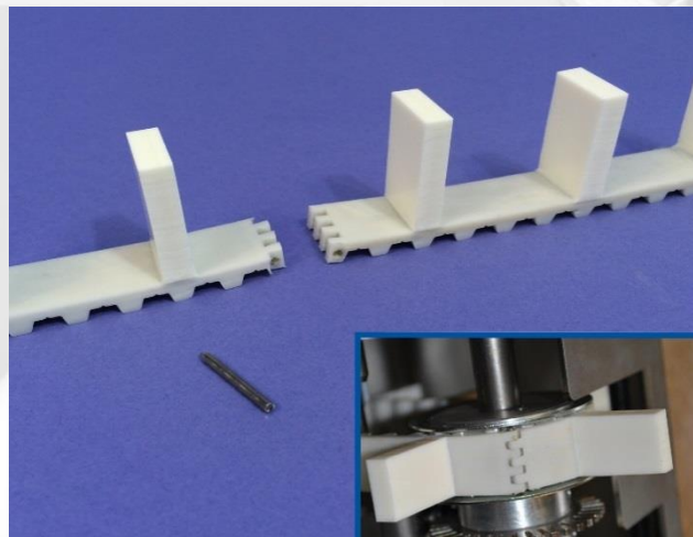
Courroie à tasseaux 16 T10 350
